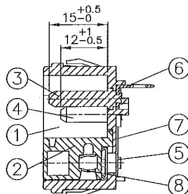
A-A 剖面
